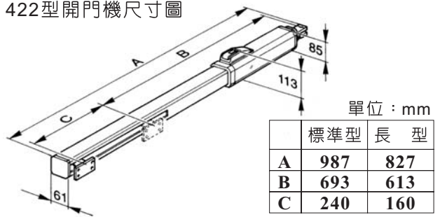
422型開門機尺寸圖
