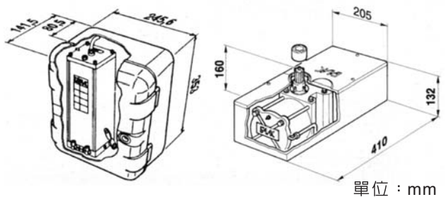
750型開門機尺寸圖
